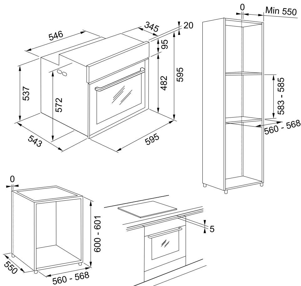
Schémas d'encastrement fours MYTHOS
