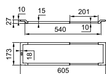
Rail télescopique 405 x 173 x 27 mm (fermé) 605 x 173 x 27 mm (ouvert)
