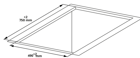
dimensions d'encastrement
