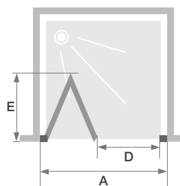
Supra S - profilé chromé
