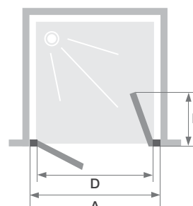
Supra 2P - profilé blanc
