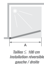
Smart Design Solo P - profilé gris noir grainé
